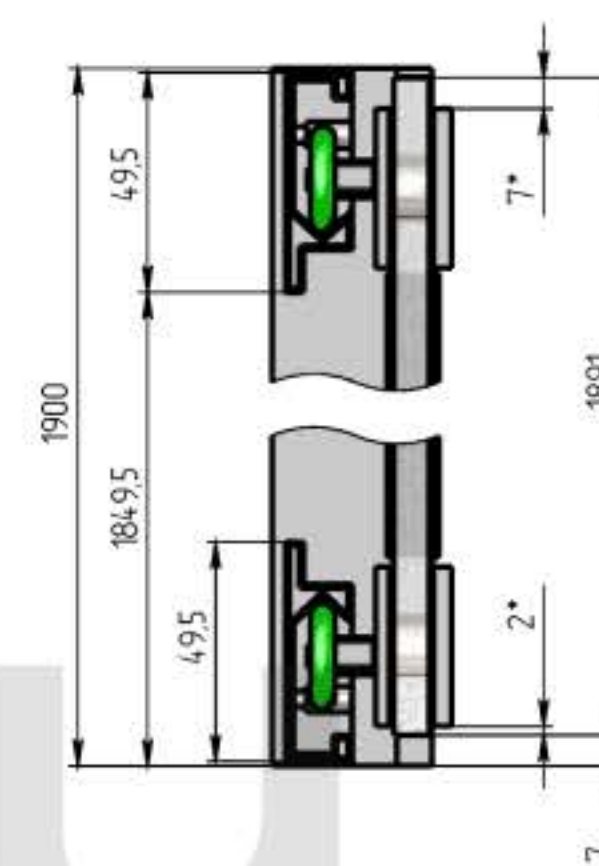
B-B (1 : 2)
